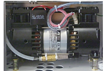
エアポンプ
